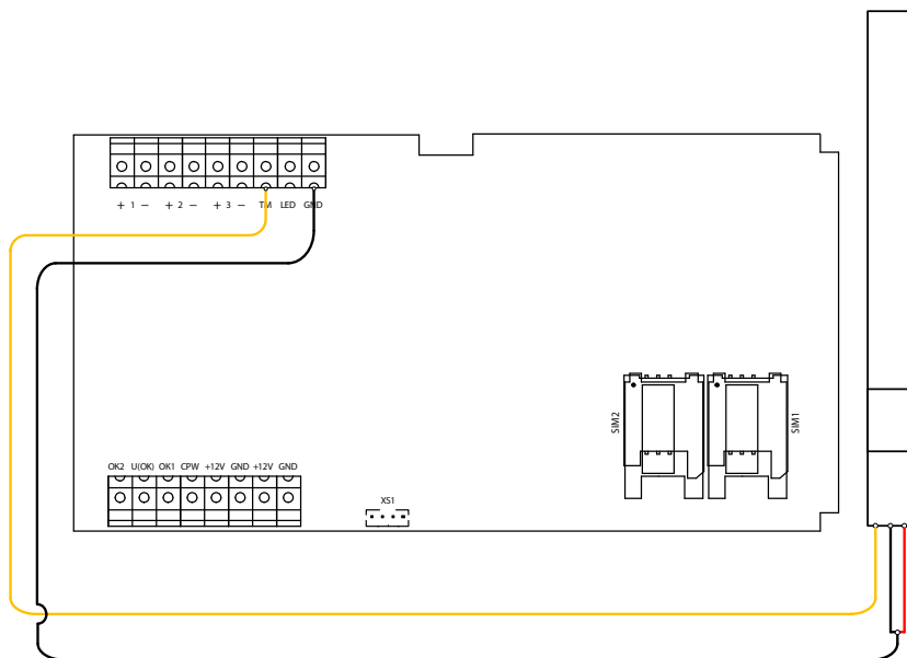
Рисунок 15. Схема подключения датчика температуры
