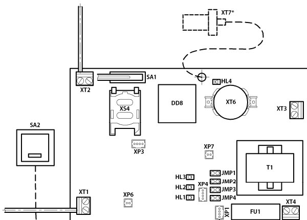
Рис. 1. Расположение устройств на печатной плате «Контакт-GSM 14»
